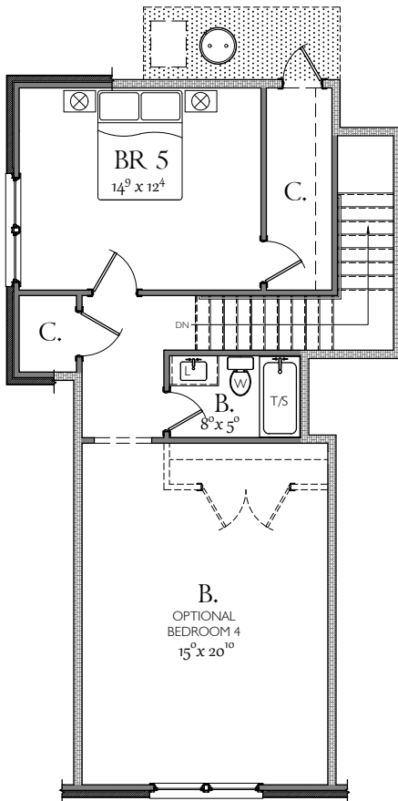
OPTIONAL BONUS -II
